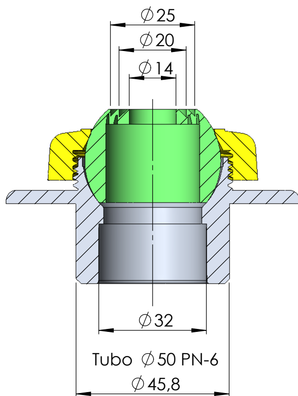
SECCIÓN B-B
